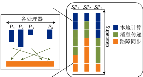
图 2 基于 BSP 模型的迭代作业执行阶段
